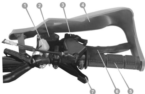
Рисунок 3.5.1. Блок перемикачів правий SP150-5
