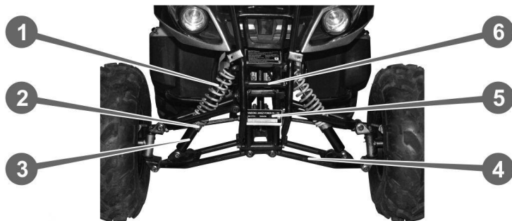
Рисунок 7.9. Передній міст
