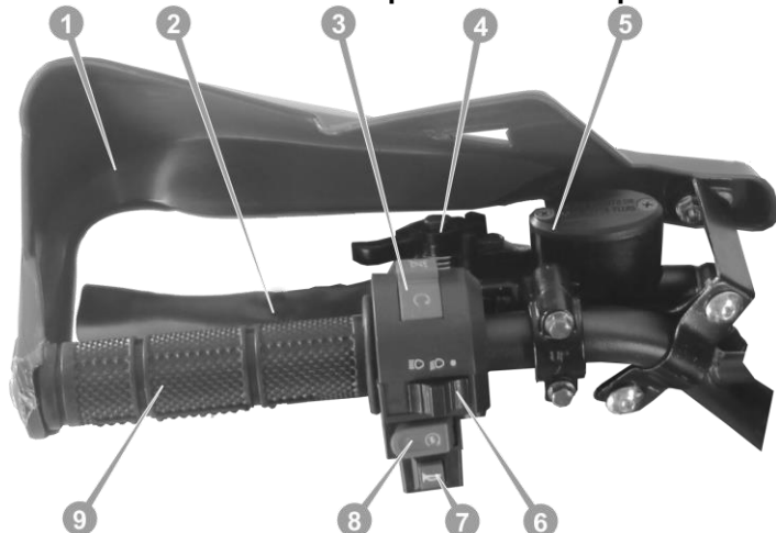
Рисунок 3.4. 1. Блок перемикачів лівий SP150-5
