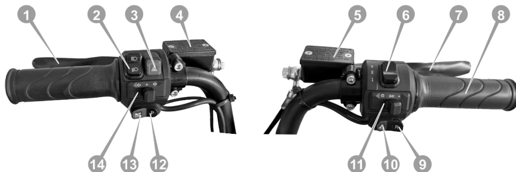
Рисунок 2.4. Блоки керування на рукоятках керма.
